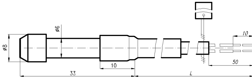
Рисунок Б.1 – ТСП-0196-21
