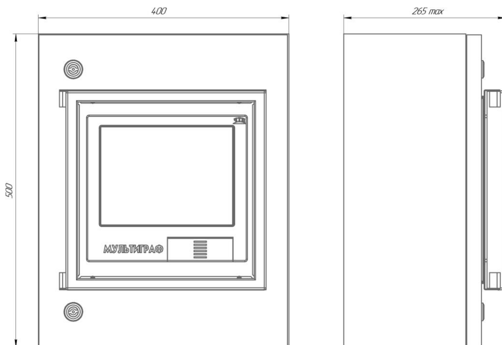
Рисунок В.4 – Габаритные размеры прибора «Мультиграф» щитового исполнения (опция Д)
